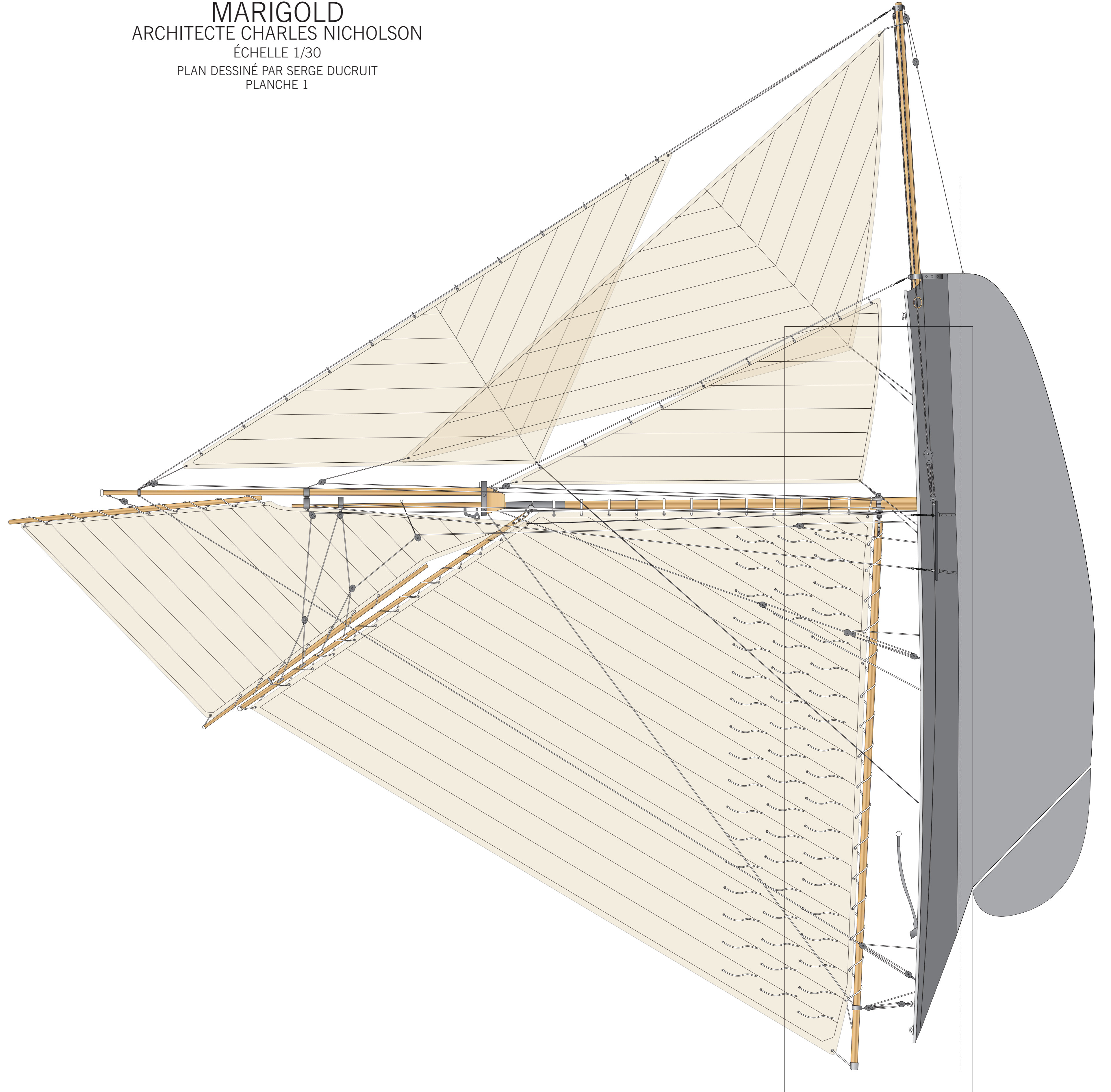
PLAN DE VOILURE AU 1 /50
